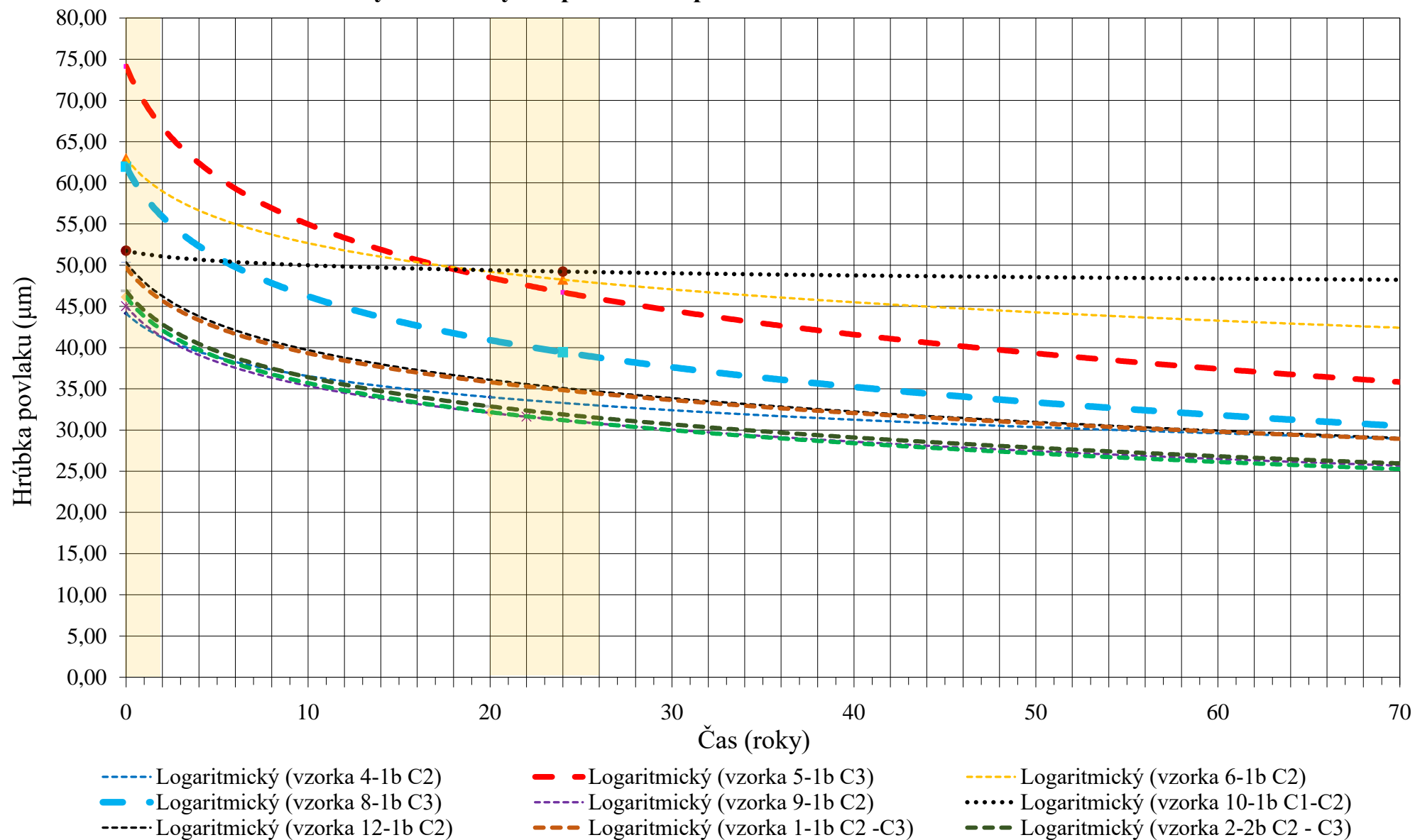
Príloha 5A Úbytok hrúbky Zn povlaku na povrchu drôtov vzoriek v kontakte s atmosférou - EV&RB
