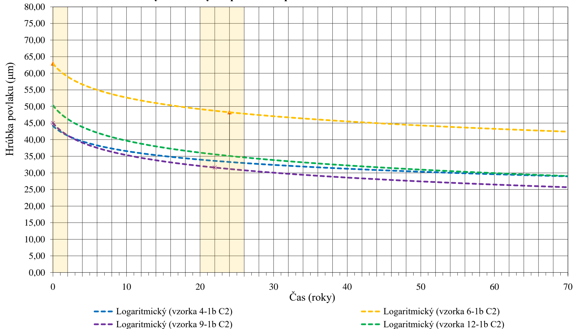
Príloha 5B Úbytok hrúbky Zn povlaku na povrchu drôtov vzoriek v kontakte s atmosférou C2 EV&RB
